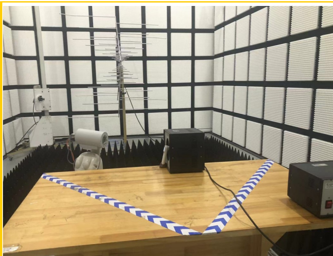
Mode 2
