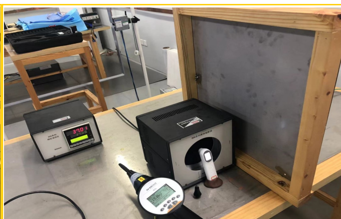
Mode 2
